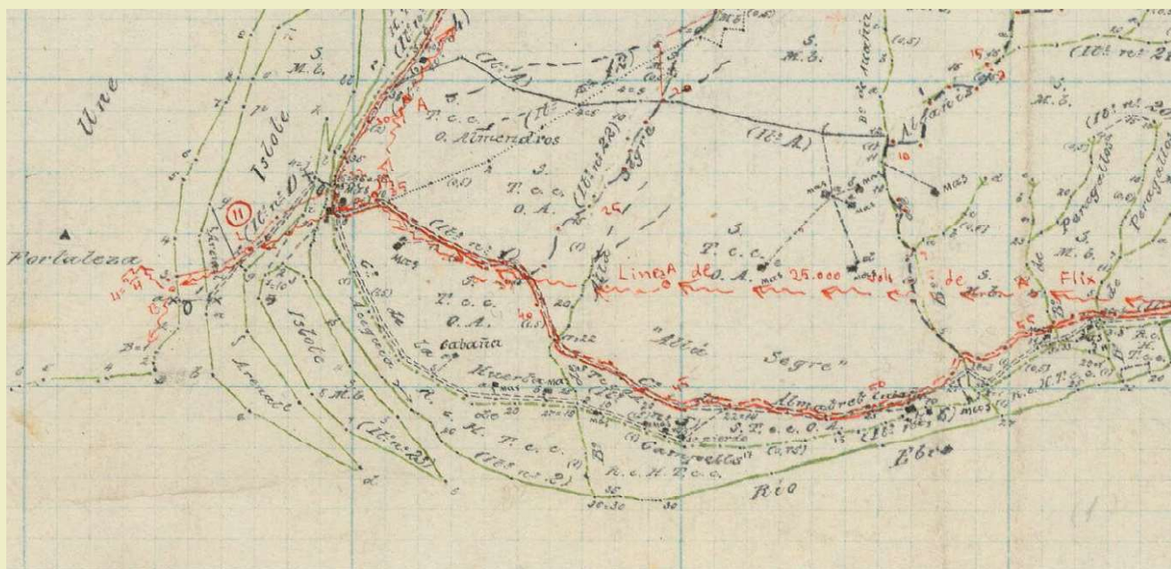
Tram final de la sèquia de la Granja d'Escarp, Campells i Della Segre. Font: IGN, Minutes municipals.
